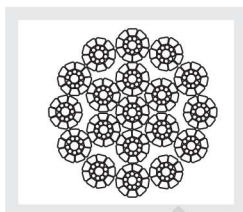
(5) 19 × 19(SL), CMP
