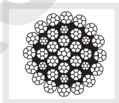
(6) 35 × 7(WA) CMP
